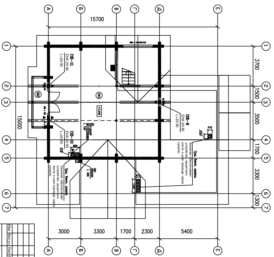
План третьего этажа М 1:100
