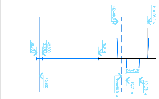
Пьезометрический график
