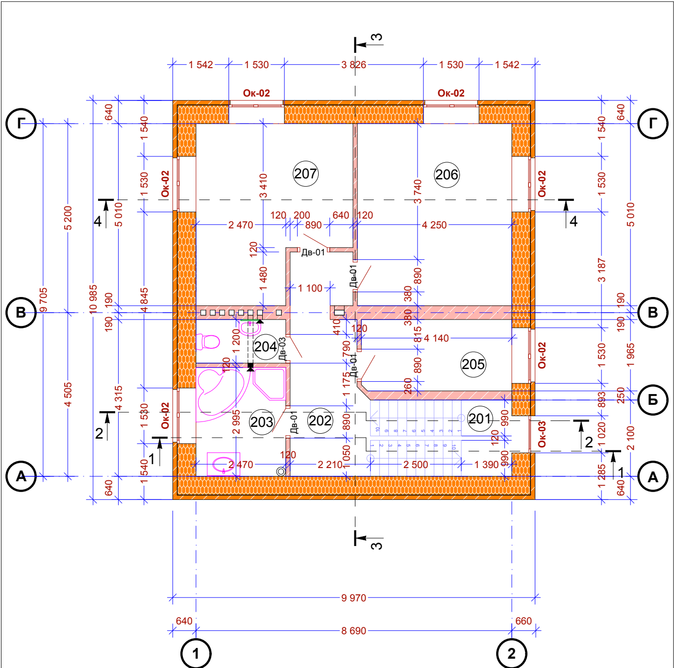
Экспликация помещений
